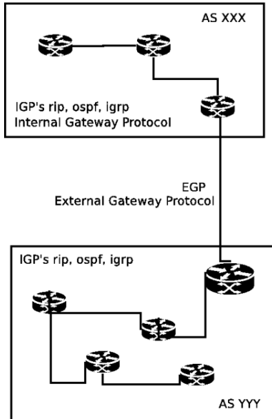
Figure 65.1. Système Autonomes
