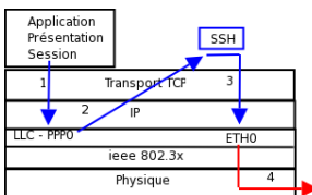
Figure 14.2. Schéma du dialogue
