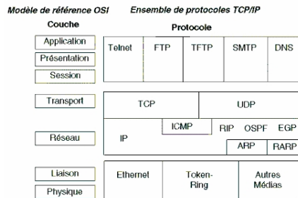
Figure 1.3. Protocoles TCP/IP et OSI
