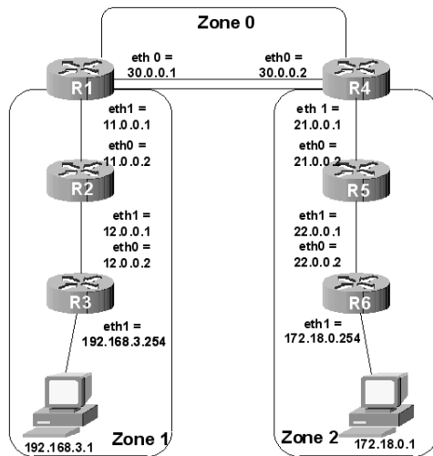
Figure 68.5. Topologie de travail
