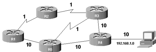
Figure 68.1. Exemple de topologie
