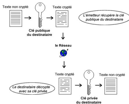
Figure 23.2. Confidentialité
