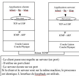
Figure 1.5. Modèle client/serveur
