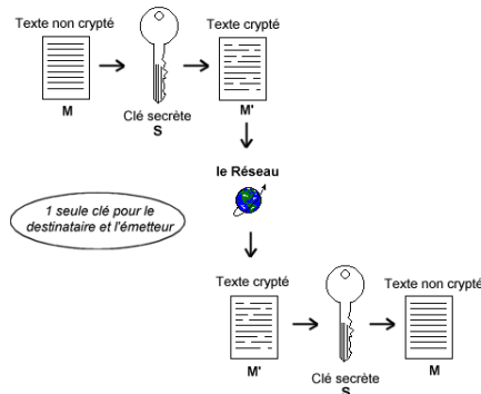
Figure 23.1. Chiffrement symétrique
