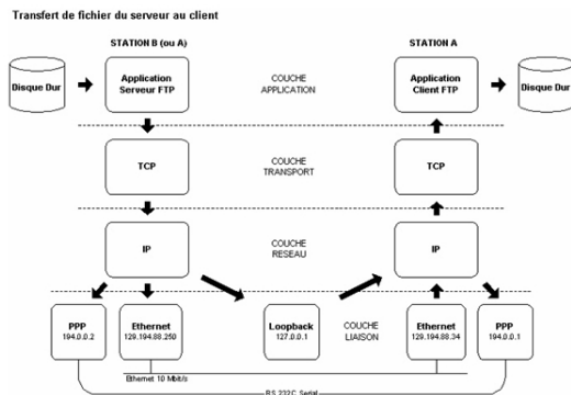
Figure 1.5. Modèle client/serveur
