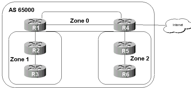
Figure 69.2. Un AS découpé en zones OSPF
