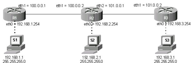
Figure 66.4. Topologie pratique
