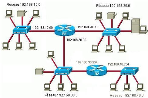
Figure 6.4. schéma de réseau 2
