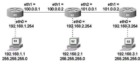
Figure 67.1. Topologie du réseau
