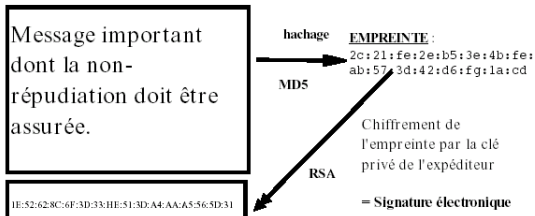
Figure 23.4. Signature électronique
