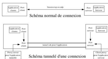
Figure 13.2. Schéma du fonctionnement
