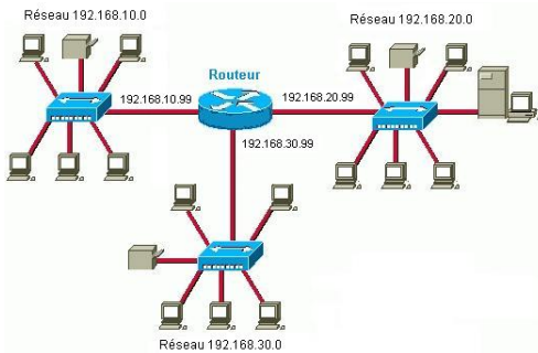
Figure 6.2. schéma de routage
